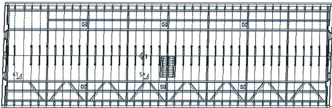
Obr. S47 – Pôdorys krovu s vyznačením polohy jednotlivých fotografií
