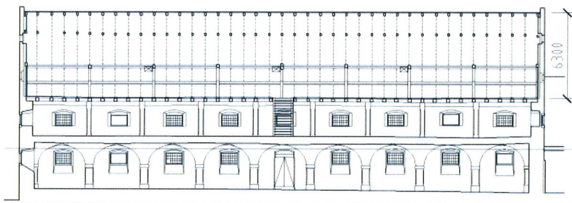
Obr. S48 – Pozdĺžny rez sýpkou
