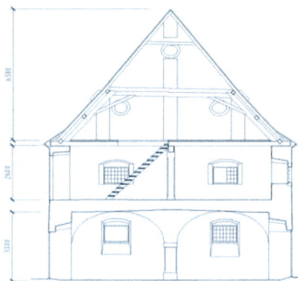
Obr. S2 – Priečny rez objektom sýpky s vyznačením jednotlivých výškových rozmerov
